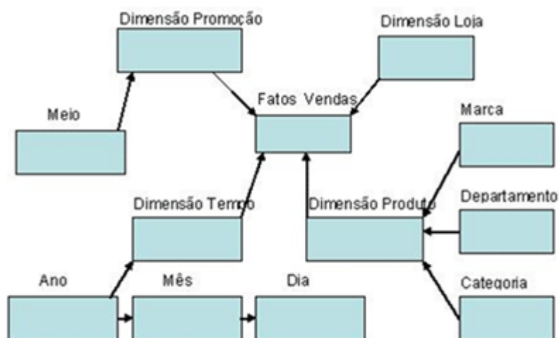
Figura 3: Modelo Snowflake
